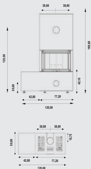
ARCHI CERAM TRI-VISION 503 Dimensions (L x H x P) : 120 x 169,8 x 50 cm
