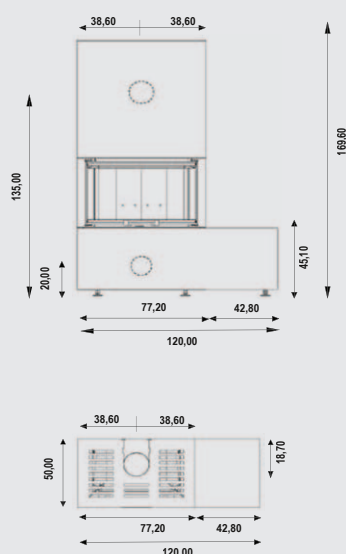
ARCHI CERAM TRI-VISION 502 Dimensions (L x H x P) : 120 x 169,8 x 50 cm
