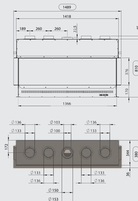
ELIUM 1500 TRI-VISION Dimensions (L x H x P) : 148,9 x 81 x 38 cm
